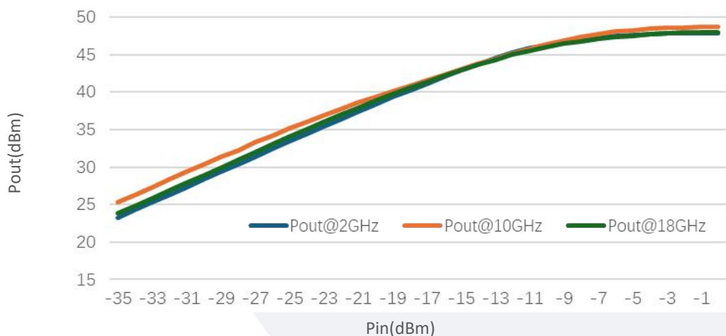
Pout@Pin
