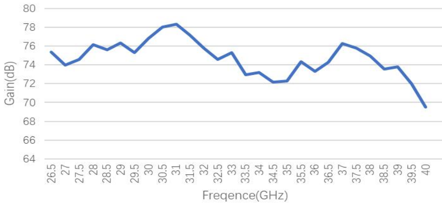
SSG@Pin=-45dBm
