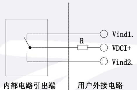
电子式指示灯电路接线图
