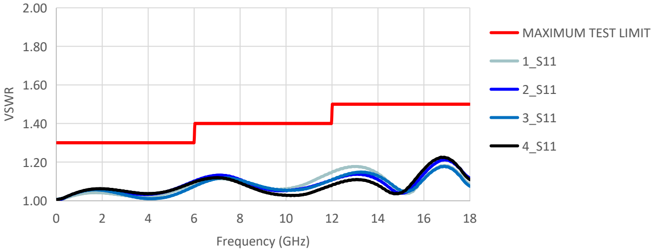
VSWR
