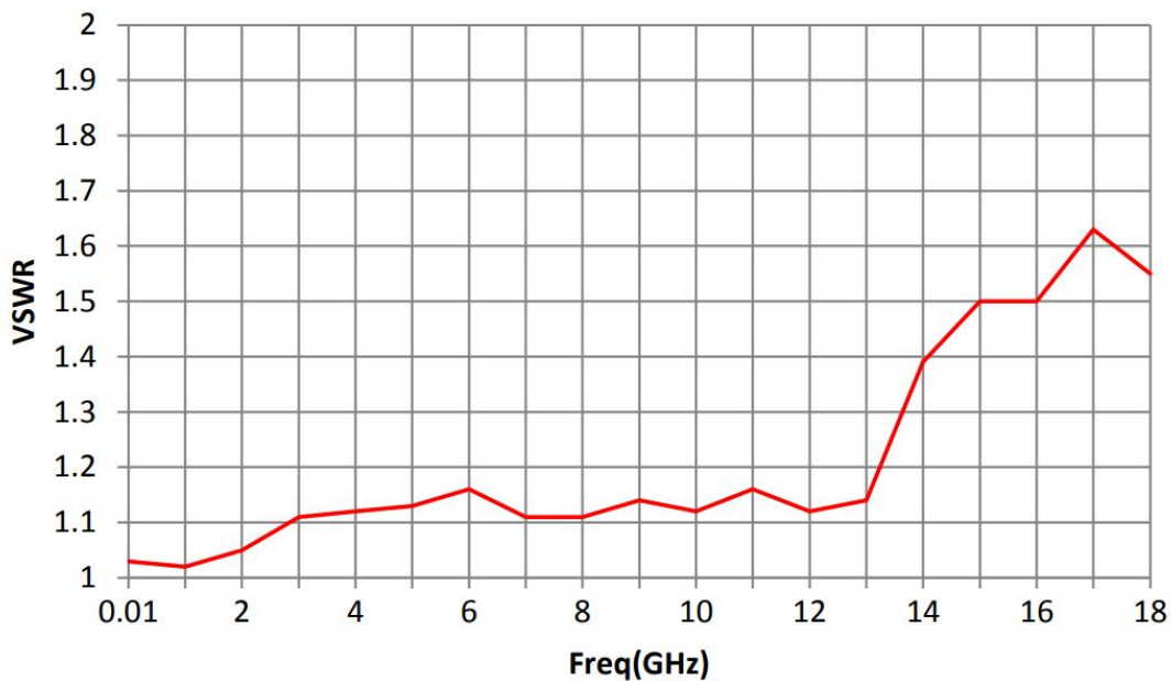
驻波比 VS 频率
