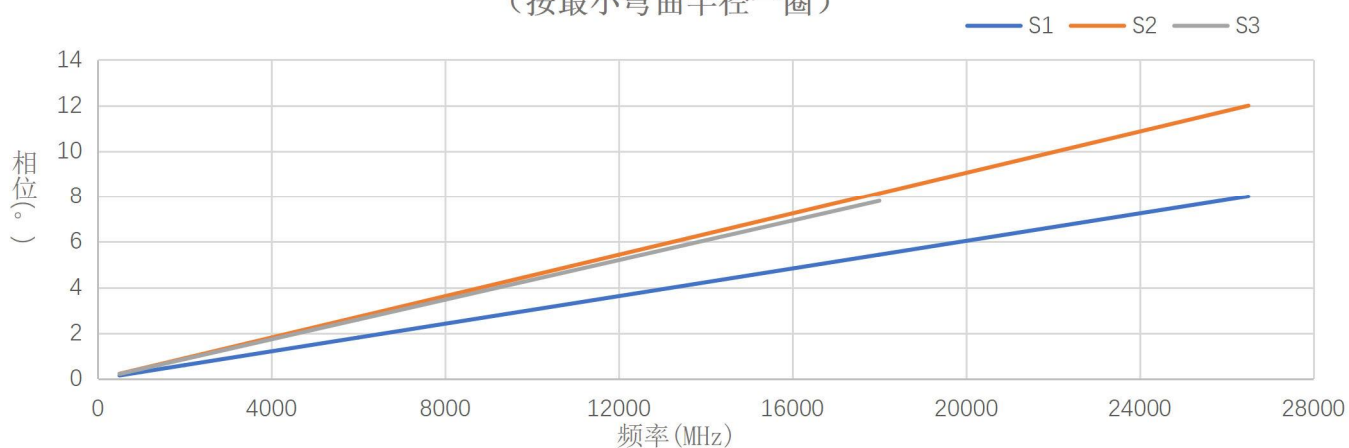
机械相位稳定性 (按最小弯曲半径一圈)
