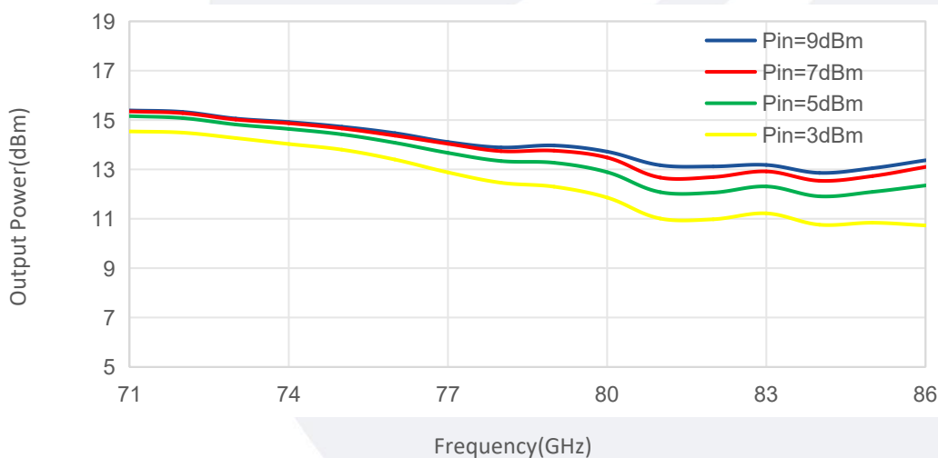
Output Power@Pin
