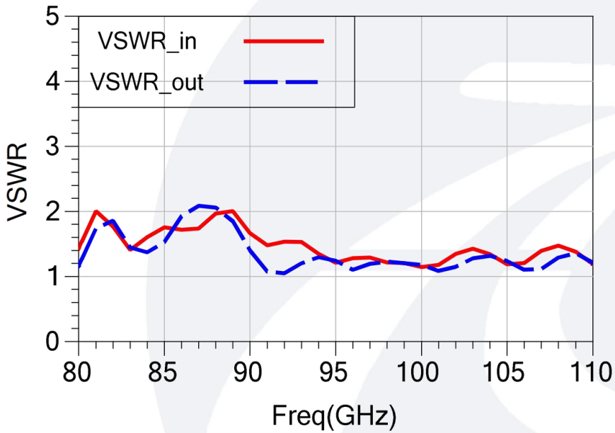
输入/输出驻波 vs. 频率
