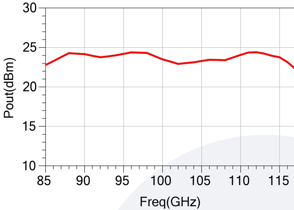
饱和输出功率 vs. 频率 @ P_{in}=14\text{dBm}
