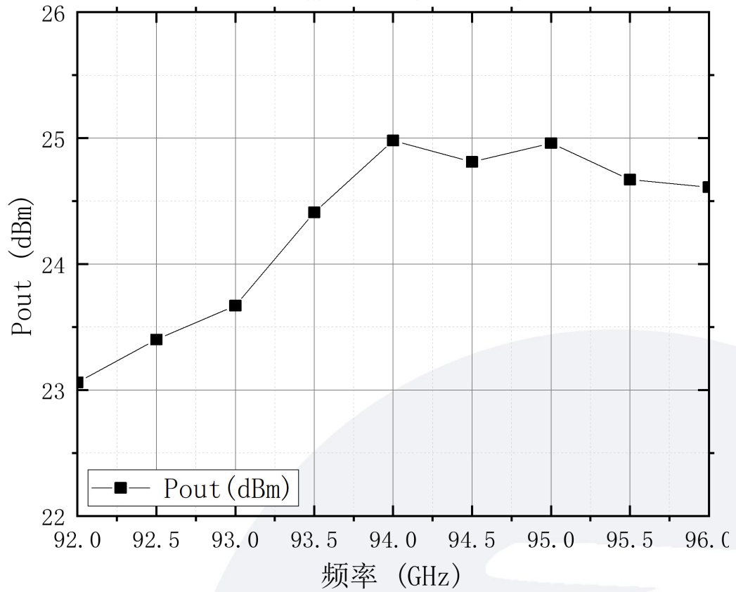
输出功率VS频率
