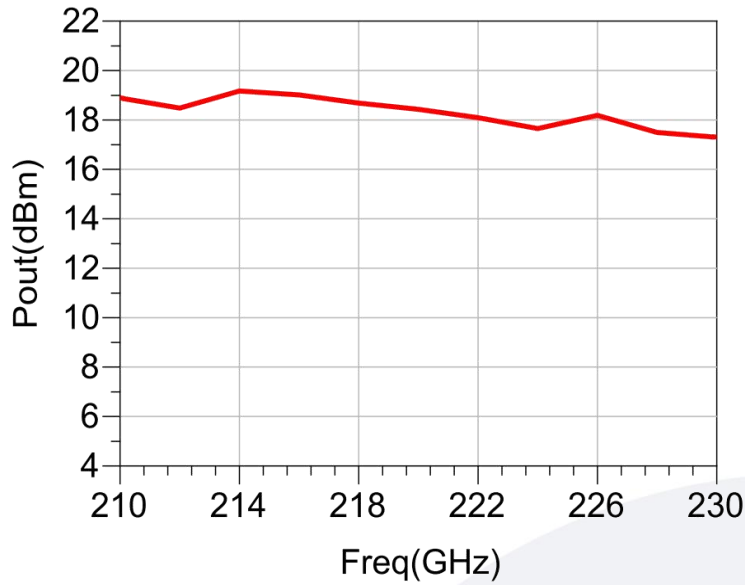
饱和输出功率 vs. 频率 @ Pin=5dBm
