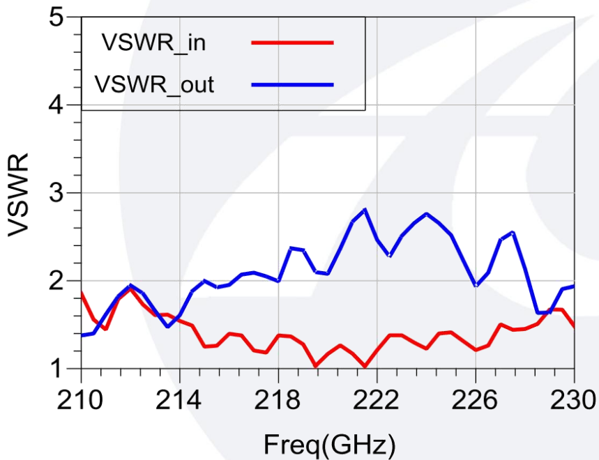
输入/输出驻波 vs. 频率
