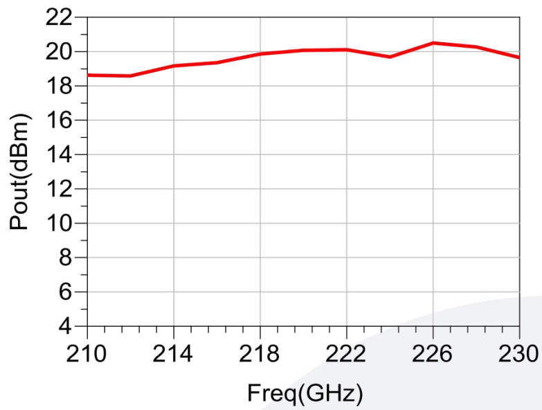
饱和输出功率 vs. 频率@Pin=15dBm
