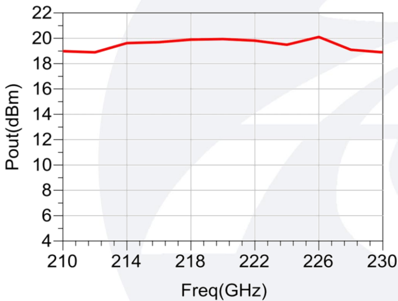
饱和输出功率 vs. 频率 @ Pin=10dBm
