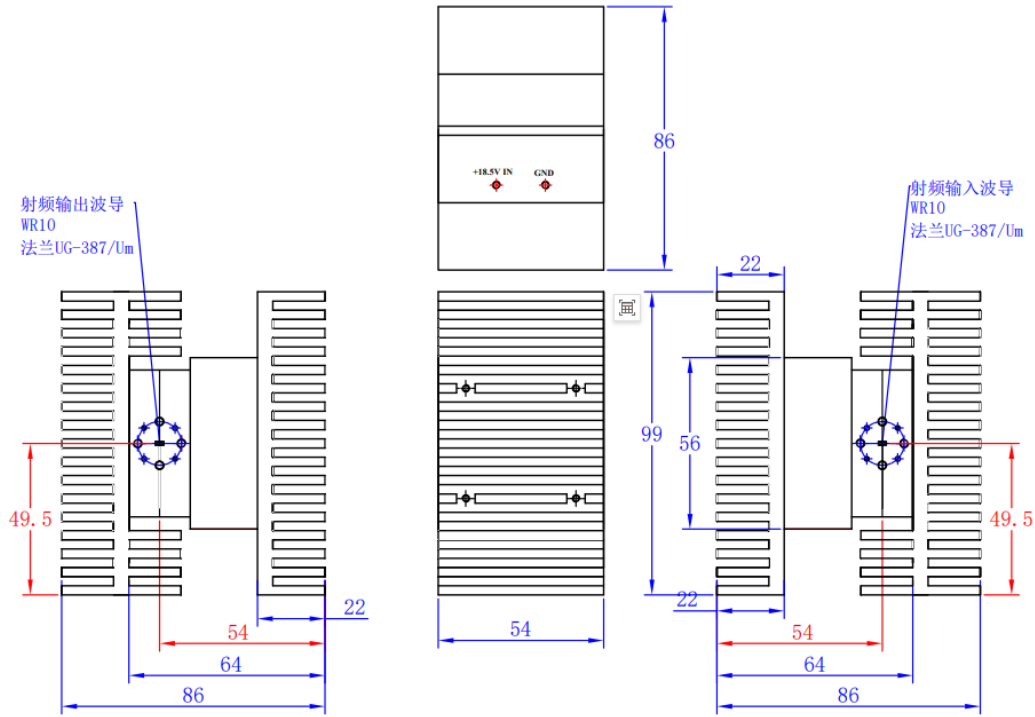
92-96GHz 30dBm 功放外形图
