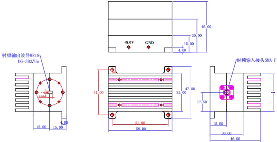
40-60GHz 15dBm四倍频器外形图
