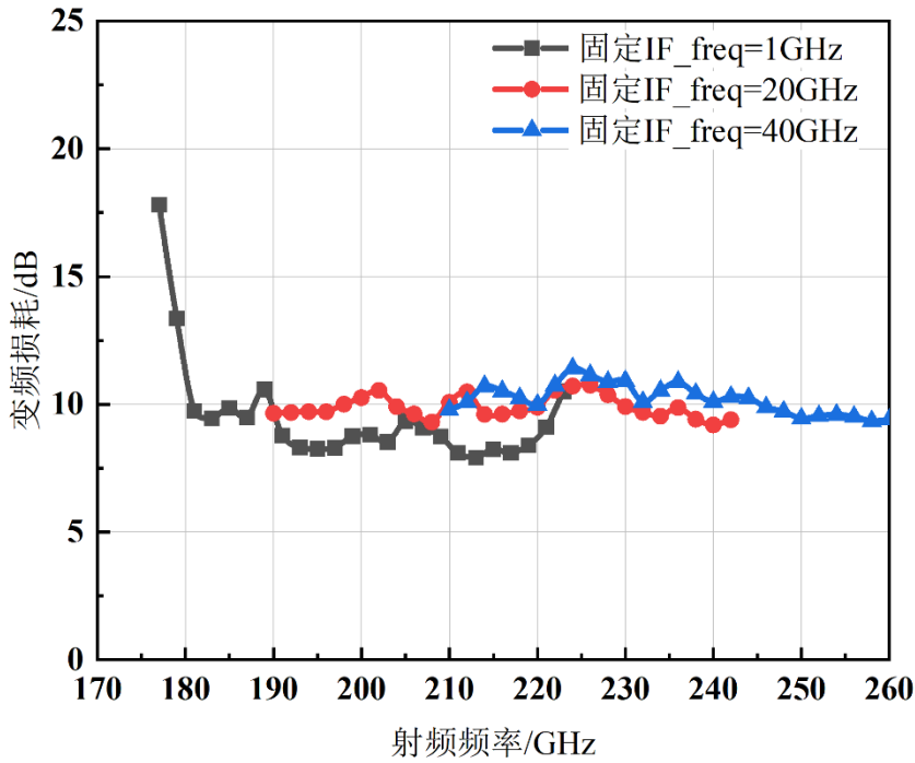
变频损耗VS频率
