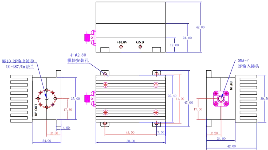
75-110GHz 20dBm六倍频器外形图
