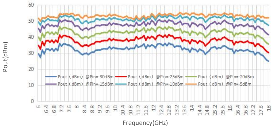
Pout@Pin
